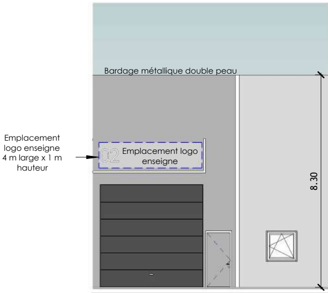
3 - FAÇADE LOT N° 02
