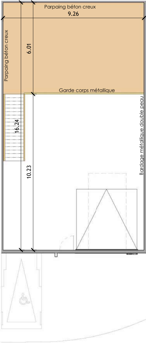
1 - LOT N° 09 - R+1
