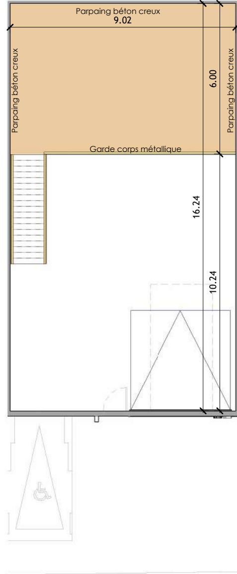
1 - LOT N° 05 - R+1
