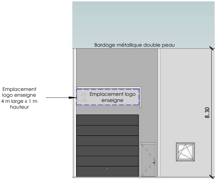
3 - FAÇADE LOT N° 12
