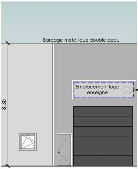
3 - FAÇADE LOT N° 03
