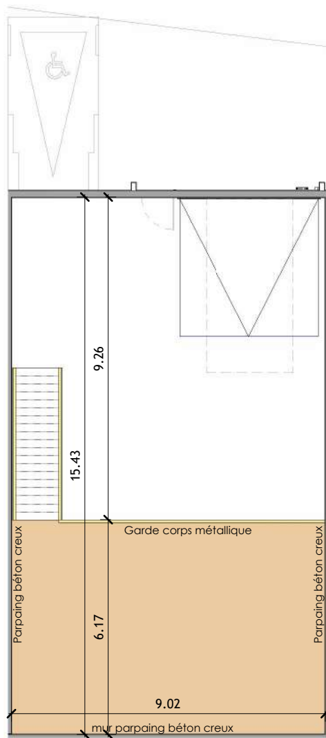
4 - COUPE LOT N° 12
