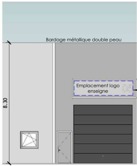
3 - FAÇADE LOT N° 05
