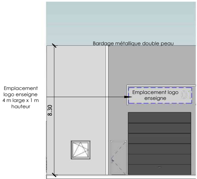
3 - FAÇADE LOT N° 01
