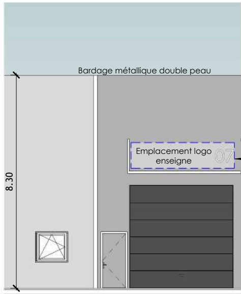
3 - FAÇADE LOT N° 07
