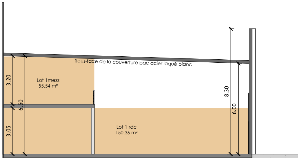
4 - COUPE LOT N° 01
