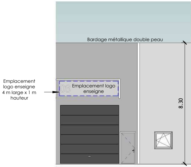
3 - FAÇADE LOT N° 08
