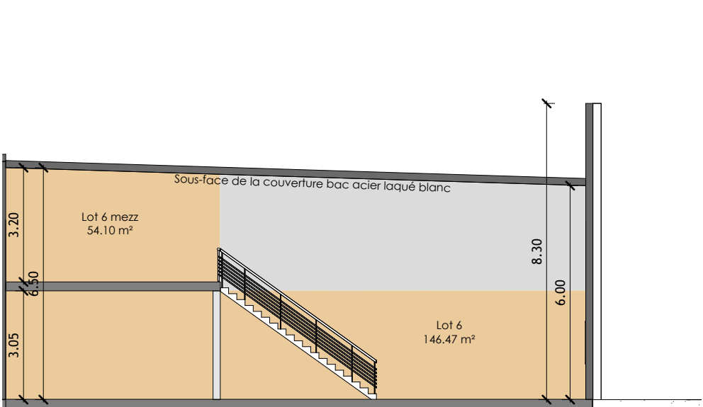
4 - COUPE LOT N° 06
